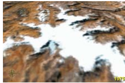
Están derritiendo los glaciares del Perú, como Qori Kalis (en la foto) debido al calentamiento global.
